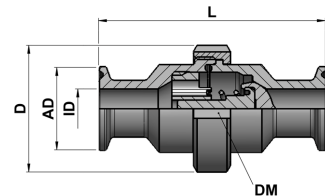
Kugelrückschlagventil mit Clamp-Stutzen
