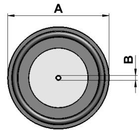
Blende mit Bohrung für TC-Verbindung DIN32676
