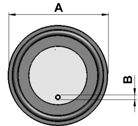
Blende mit exzentrischer Bohrung für TC-Verbindung DIN32676
