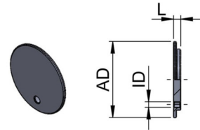
Blende mit exzentrischer Bohrung für Clamp-Anschluss DIN32676
