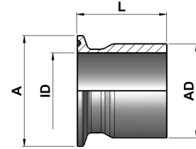
Tankanschweissklemmstutzen DIN32676
