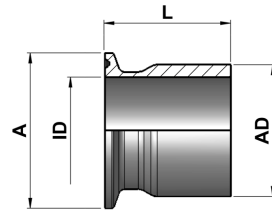
Tankanschweissklemmstutzen DIN32676
